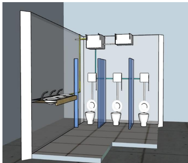
Figura 14 – Perspectiva Frontal 3D.
